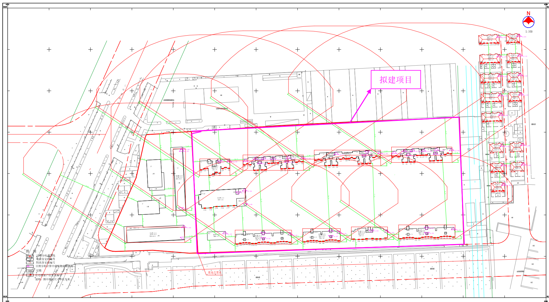
图 3.3-4 拟建项目大寒日日照分析图
